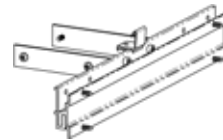
Blendenaufnahme stirnseitig
