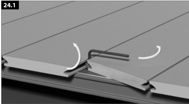
Inbus (4 mm) einsetzen und um 90° drehen.
